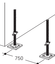
Obrázek A-1: Varianta založení na samostatných podložkách
