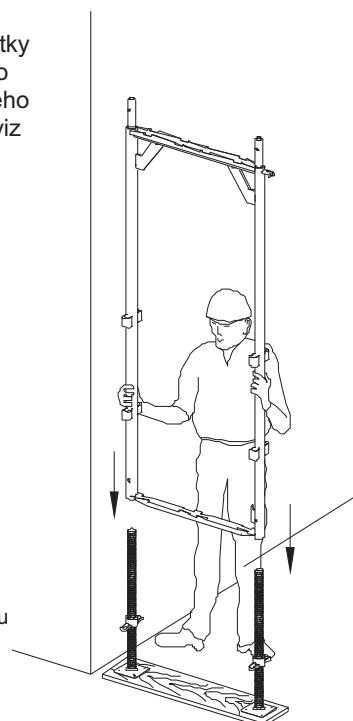
Obrázek B: Nasazení rámu na stavitelnou patku
