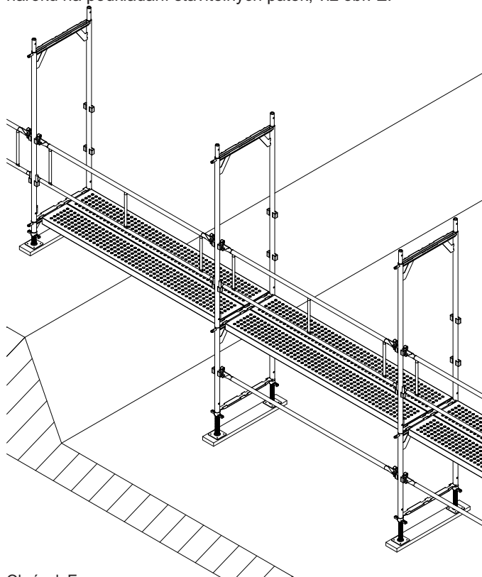
Obrázek E: Založení na skloněném terénu
