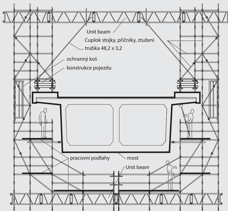
Sanační lávka
