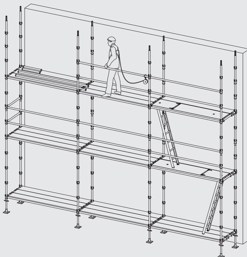
Postup montáže vyšších pater
