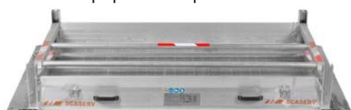
Lávka se sklopeným zábradlím připravena k přepravě
