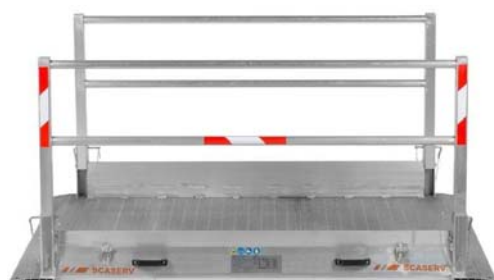
Lávka se zajištěným zábradlím připravena k použití
