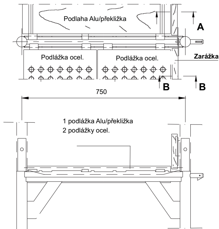
PŮDORYS
