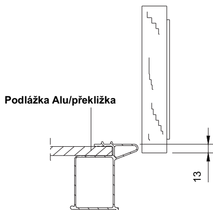
ŘEZ A-A
