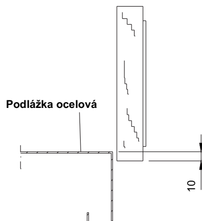
ŘEZ B-B
