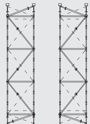
pohled čelní
