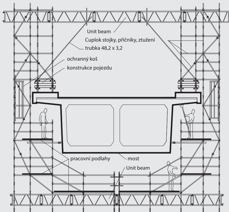
Sanační lávka
