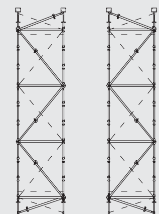
pohled boční
